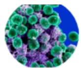
Staphylococcus pasteuri
